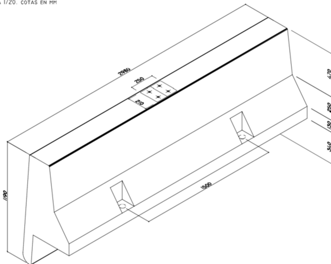
IMP03. IMPOSTA DE BARRERA: 868 KG/ML ESCALA 1/20. COTAS EN MM
