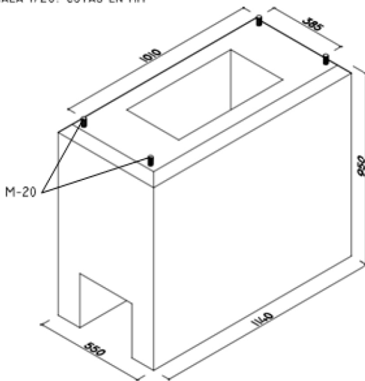
BAS004. BASAMENTO DE ARMARIO GRANDE: 110 KG/UD ESCALA 1/20. COTAS EN MM
