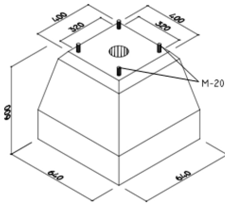
BAS0II. BASAMENTO DE MÁSTIL DE MANDO LOCAL 490 KG/UD ESCALA 1/20. COTAS EN MM
